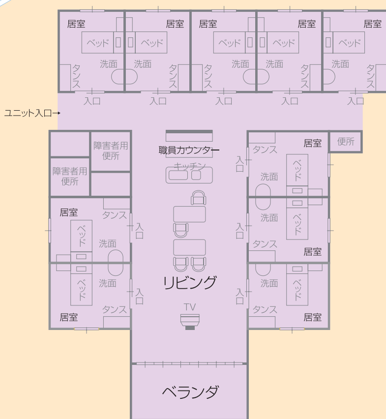
ユニットのイメージ平面図
